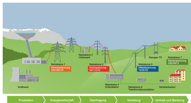
Der Weg des Stroms vom Kraftwerk zum Verbraucher
